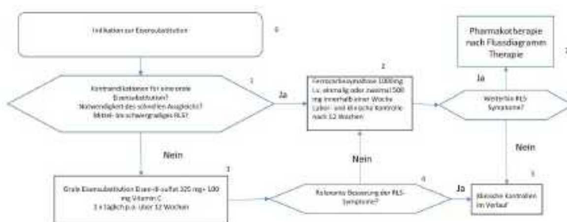
Abbildung 1: Algorithmus Eisensubstitution
